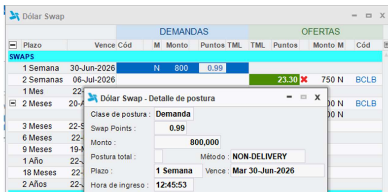
Ilustración 13 Detalle Postura
