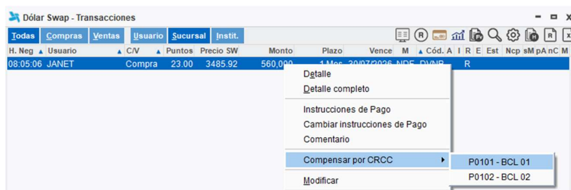
Ilustración 70 Opción Compensación
