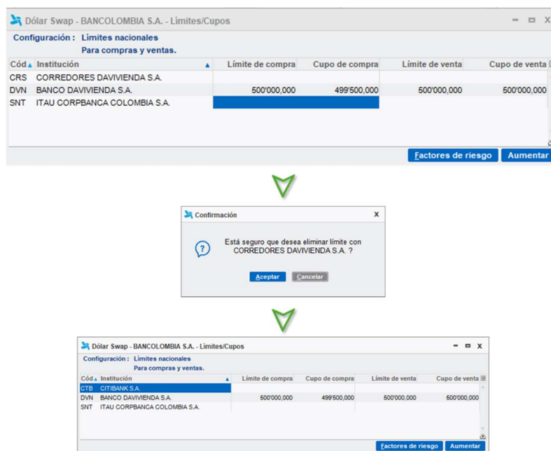
Ilustración 30 Ventana Cupos
