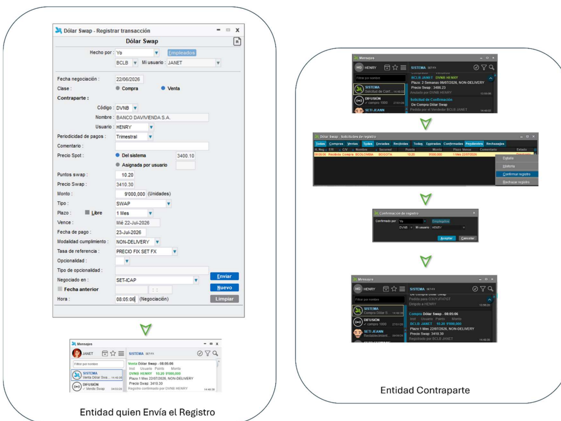
Ilustración 18 Ejemplo Registro
