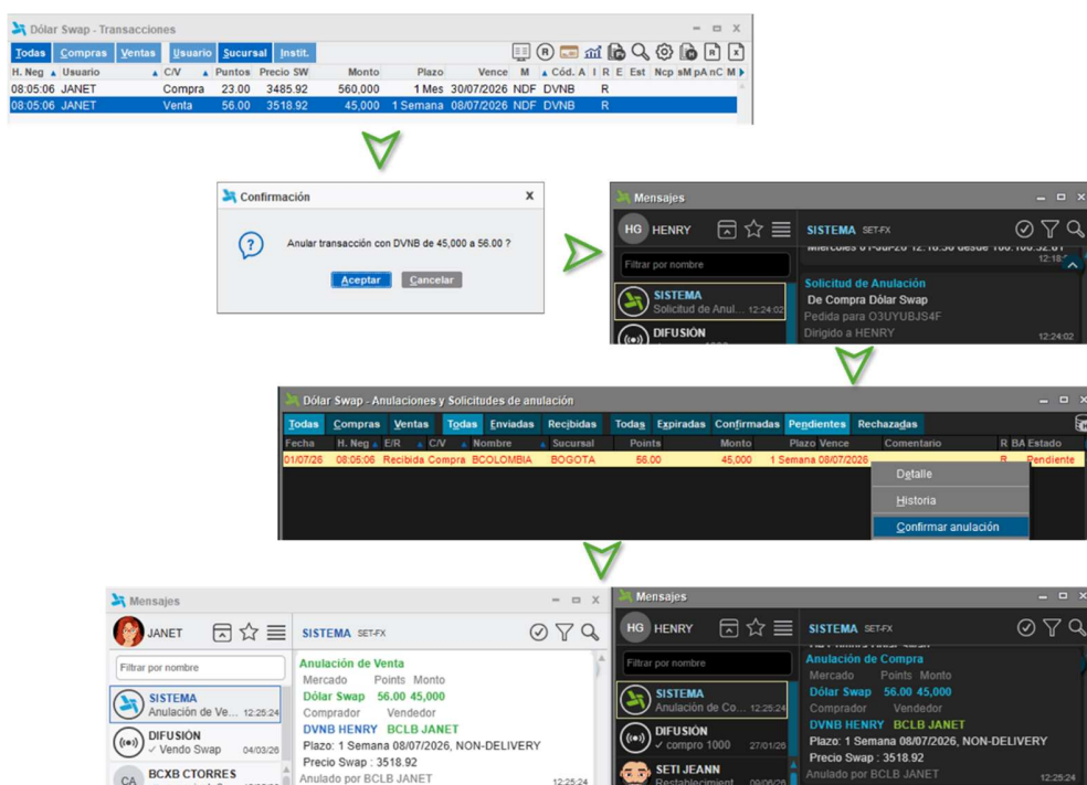
Ilustración 69 Ejemplo Anulación
