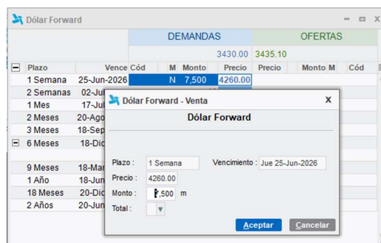
Ilustración 9 Agredir Postura
