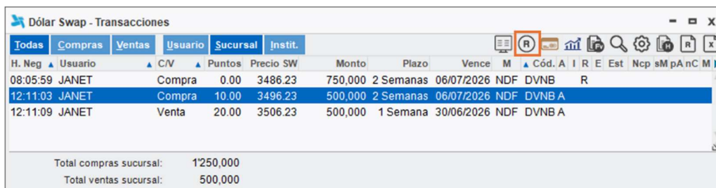
Ilustración 14 Botón Registro
